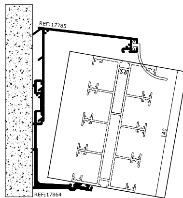
- TECHO FIJO 4 CARRILES
