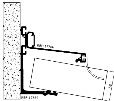
- TECHO FIJO PANEL 52 MM
