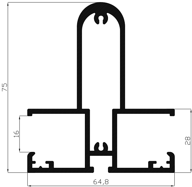
PERFIL H 16 70520 Medida 6.5 metros
