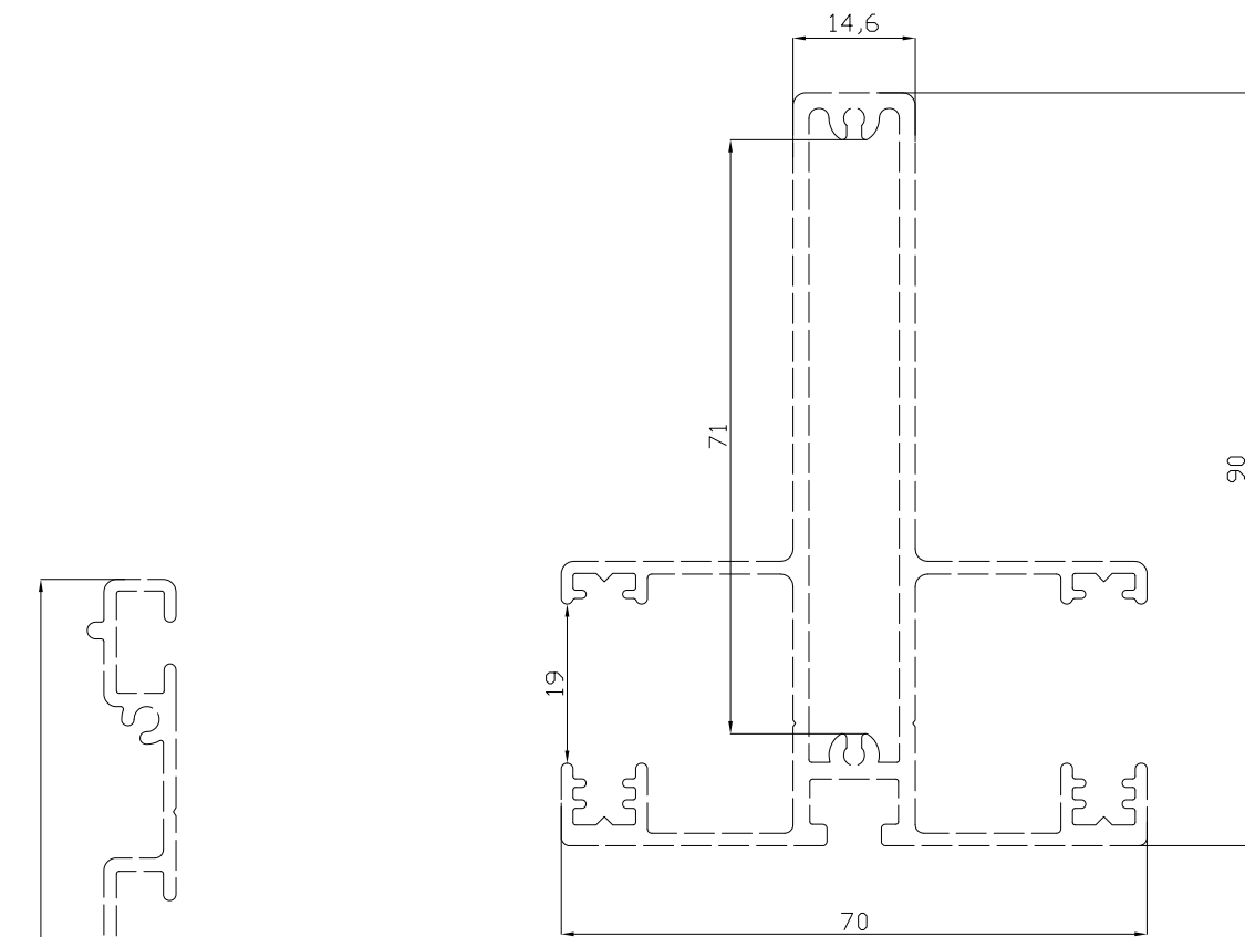
PERFIL REFORZADO PARA TECHOS FIJOS
