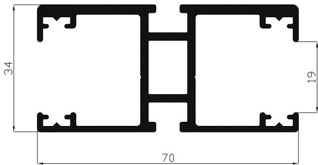
ACOPLE VIGA 17922 Medida 6.5 metros
