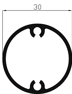
REDONDO ATURROSCABLE DE 30 MM 55095 Medida 6.5 metros
