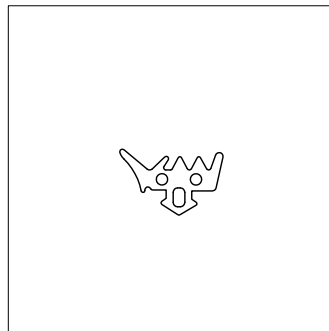
Junta para hoja de vidrio. (Perfil 18257) REF: 25167
