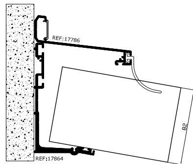
- TECHO FIJO PANEL 82 MM
