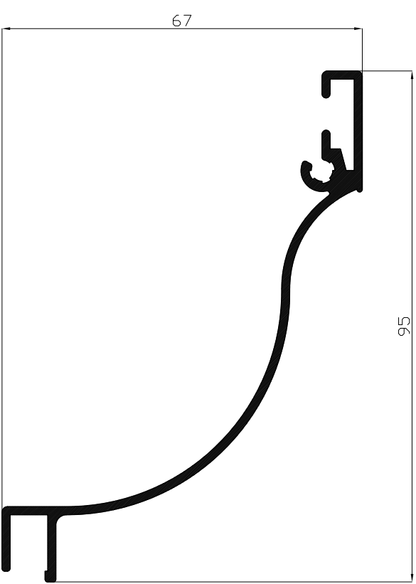
REMATE CANAL CURVO 20299 Medida 6.5 metros
