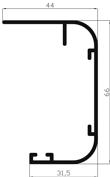
EMBELLECEDOR 52 MM 70504 Medida 6.5 metros
