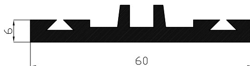
PERFIL UNIÓN PANEL 70521 Medida 6.5 metros
