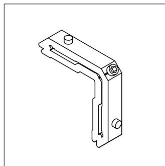
Escuadra exterior marco 65 Hoja acristalar REF: 4910
