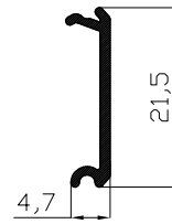
TAPETA VIGA 15654 Medida 6.5 metros
