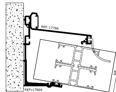
- TECHO FIJO 2 CARRILES
