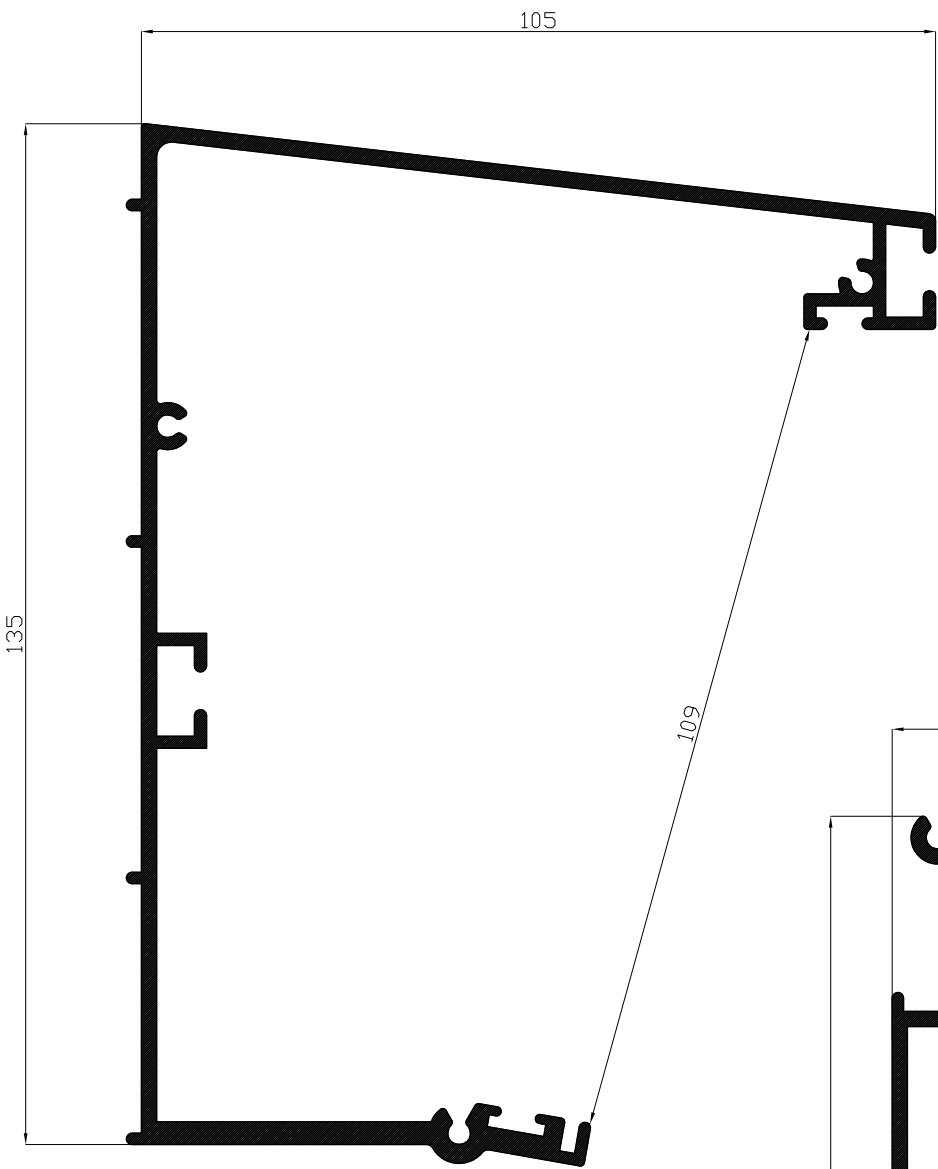
SOPORTE COBIJA 20298 Medida 6.5 metros
