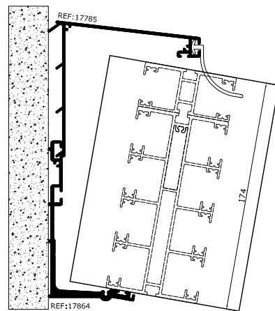
- TECHO FIJO 5 CARRILES
