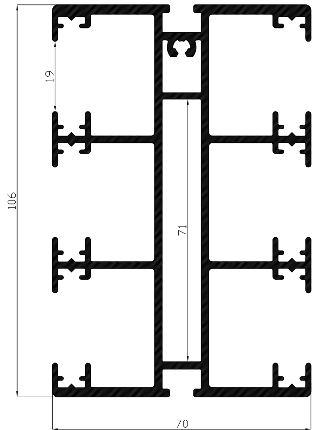
VIGA 3 CARRILES 17784 Medidas de 4.5 y 6.5 metros
