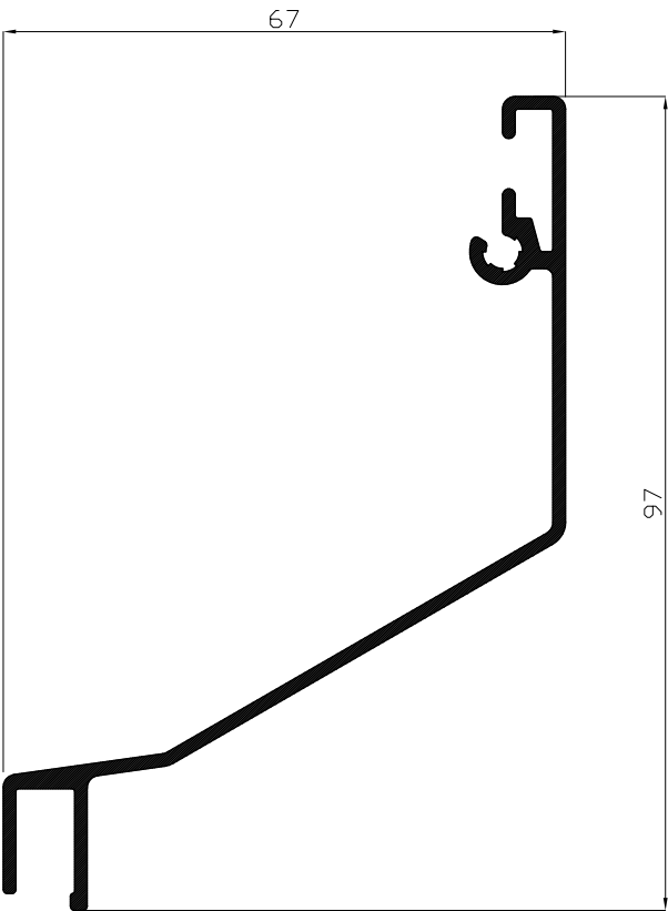
REMATE CANAL 17782 Medida 6.5 metros
