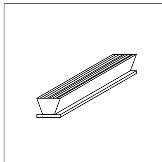
Felpudo Fin-Seal 7x11 mm (Perfil hoja cruce 17787) REF: 2061
