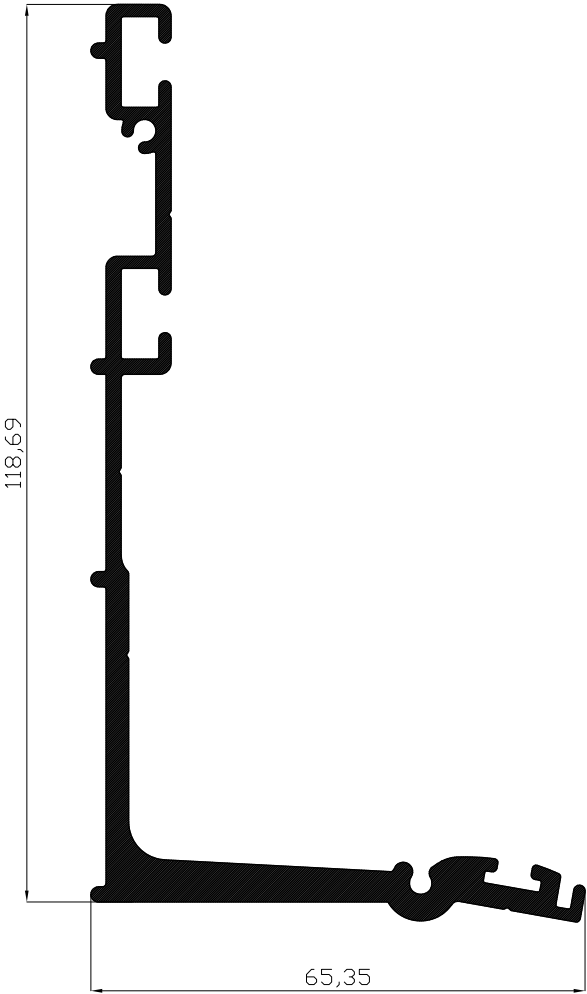
SOPORTE COBIJA 17864 Medida 6.5 metros
