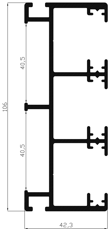
VIGA LATERAL 3 CARRILES 17920 Medida 6.5 metros
