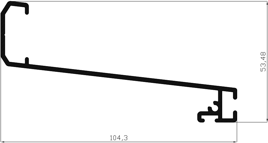
COBIJA 17786 Medida 6.5 metros
