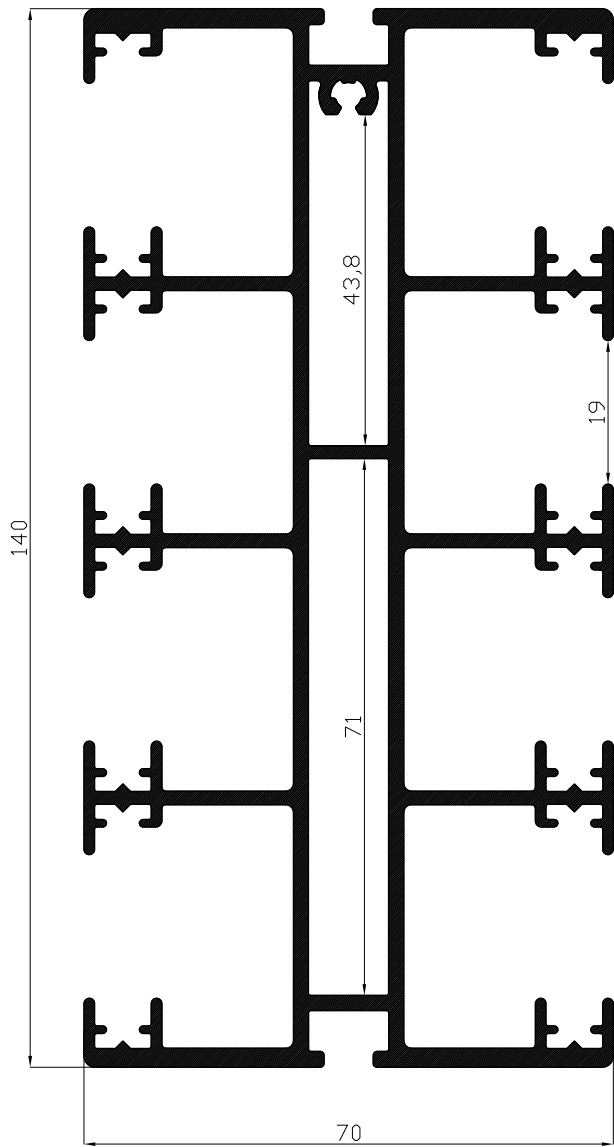
VIGA 4 CARRILES 17930 Medidas 5.5 y 6.5 metros
