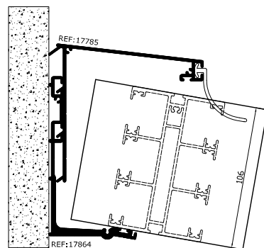
- TECHO FIJO 3 CARRILES
