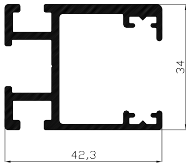
ACOPLE VIGA LATERAL 17921 Medida 6.5 metros
