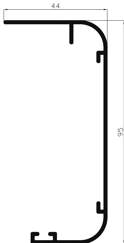
EMBELLECEDOR 82 MM 70503 Medida 6.5 metros
