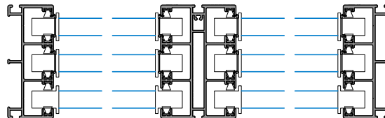
Sección Vertical
