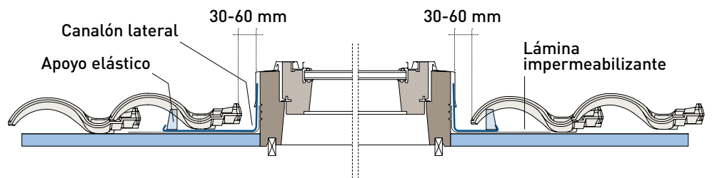
SECCIÓN TRANSVERSAL
