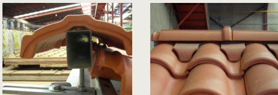
Instalación de Q01 con Teja Mixta (TG - TP)
