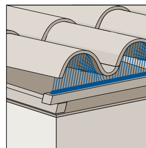
Peine de alero
