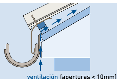
ventilación (aberturas &lt; 10mm)
