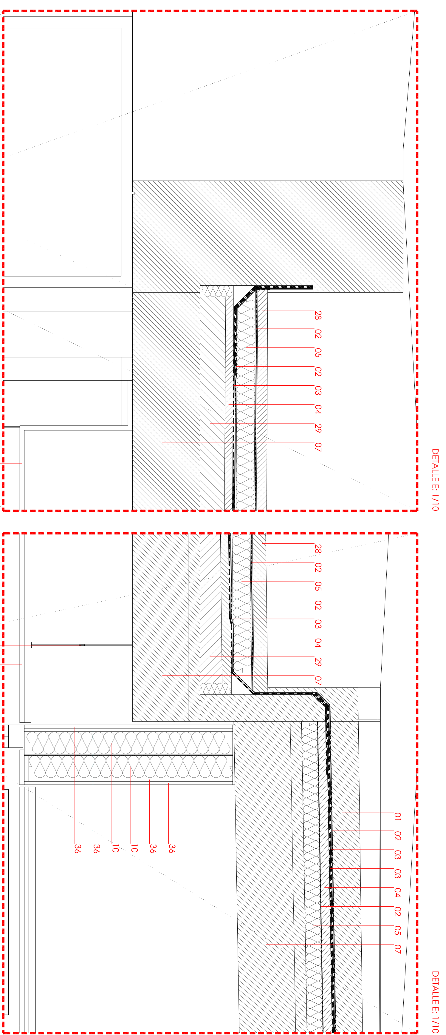
DETALLE E: 1/10
