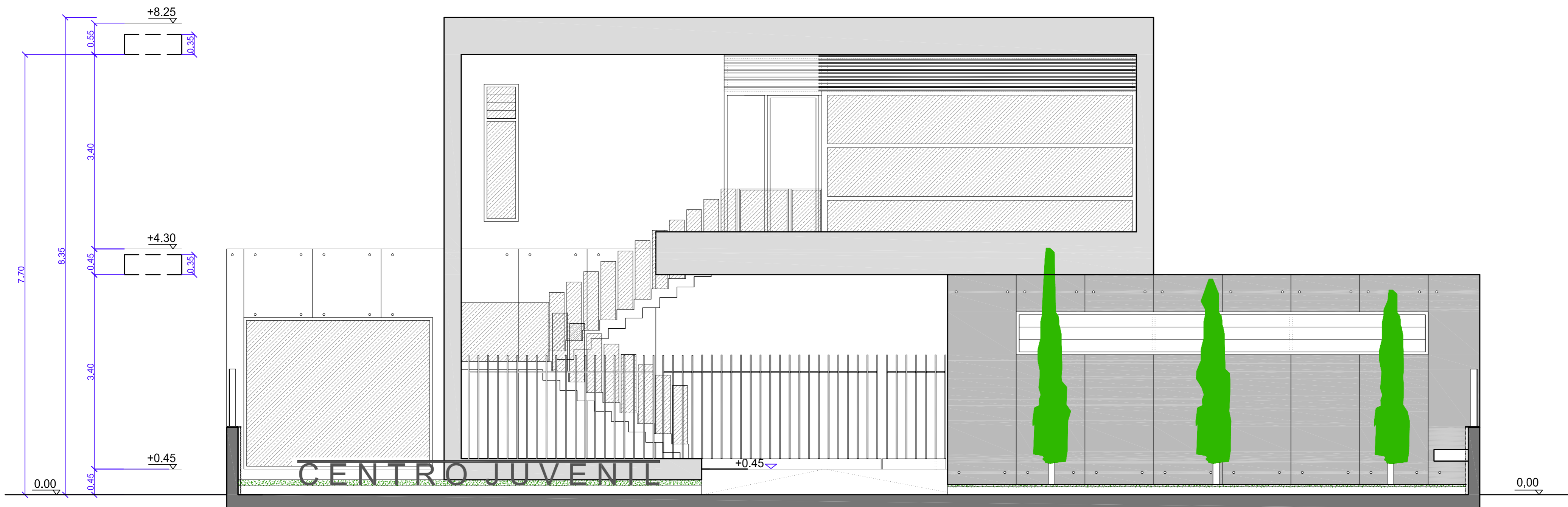
ALZADO SUR
